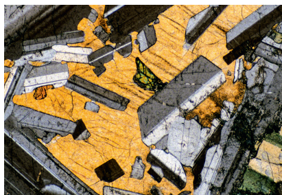
Atelier microscope : Gabbro à pyroxène. Microphotographie réalisée en lumière polarisée.
